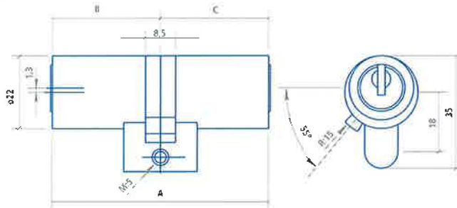
Cilindro SEA 3 / SEA 23
