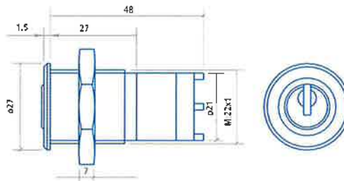
Microconmutador SEA 3 / SEA 23
